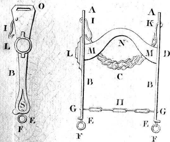
Fig. 1 re Le Mors
